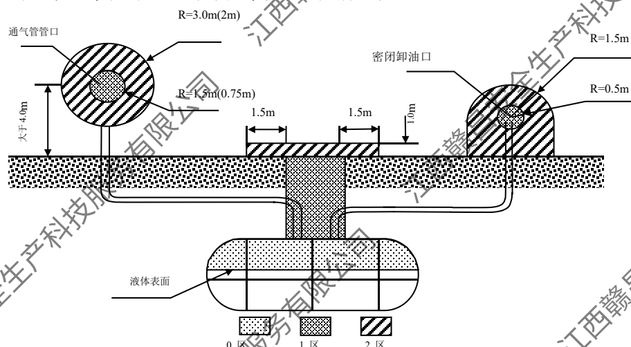
图 3-1 地下卧式油罐危险区域分布图
