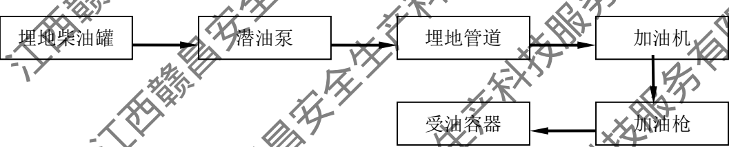
图 2.5-4 柴油加油工艺流程图示意简图
